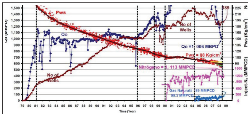
شکل ۲ | نمودار تاریخچه تولید و تزریق میدان کانتارل [۲]
