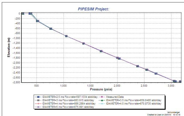
شکل ۴ | بررسی اثر تغییرات قطر لوله مغزی بر عملکرد فشار جریانی
