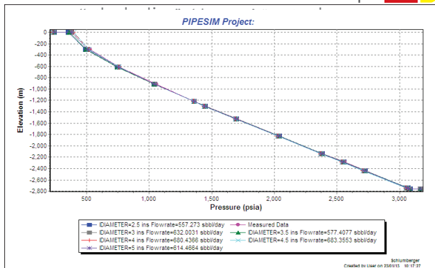
شکل ۵ | بررسی اثر تغییرات قطر لوله مغزی بر عملکرد فشار جریانی سرچاهی در عمق نصب ۱۳۰۰ متر حفار برای چاه-۲
