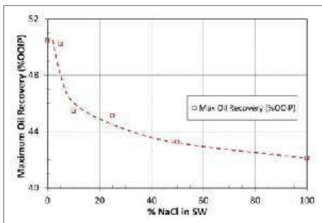
شکل ۸ | بالاترین بازده تولید نفت با استفاده از آب دریا تصحیح‌شده در غلظت‌های مختلف از NaCl در دمای 90^{\circ}C و اشباع آب اولیه ۱۰ درصد و عدد اسیدی ۰/۵ میلی‌گرم از KOH در گرم [۱۱]
