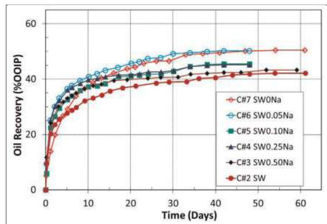
شکل ۷ | بازده تولید نفت در آشام خودبه‌خودی از سنگ چالکی اشباع از نفت برای آب هوشمند در غلظت‌های متنوع از یون Na در دمای 90^{\circ}C و اشباع آب اولیه ۱۰ درصد و عدد اسیدی ۰/۵ میلی‌گرم از KOH در گرم [۱۱]
