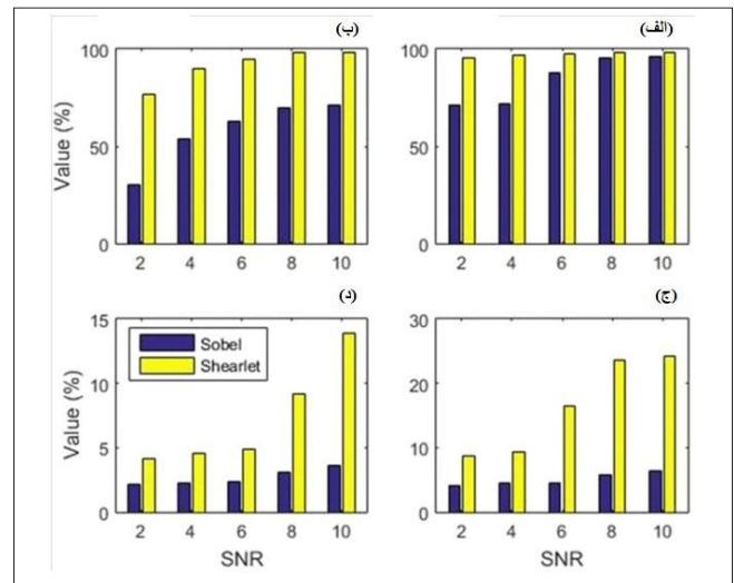
شکل ۶ | مقایسه‌ی کمی طرح‌واره‌ی شیرلت دوبعدی و پالایه‌ی سوبل با استفاده از آزمایش دسته‌بندی دودویی: الف) ویژگی (ب) دقت (ج) اندازه‌ی F-د) حساسیت برای نسبت‌های سیگنال به نوفه ۲، ۴، ۶، ۸، ۱۰ و ۱۰۰ از آنجا که عملگر کنی نتایج کیفی قابل‌قبولی ارائه نداده در محاسبه‌ی کمی از آن استفاده نشده است
