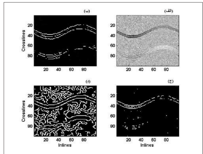
۵ شکل الف) برش زمانی از داده‌های لرزه‌نگاری مصنوعی حاوی دو کانال در زمان ۶۴۸ میلی‌ثانیه با نسبت سیگنال به نوفه ۵. ب-د) لبه‌های شناسایی شده‌ی کانال‌ها به ترتیب توسط طرح‌واره‌ی شیرلت دوبعدی، پالایه‌ی سوبل و عملگر کنی، همان‌گونه که پیداست طرح‌واره‌ی شناسایی لبه با استفاده از شیرلت‌های دوبعدی نسبت به پالایه‌های سوبل و کنی در مرزهای کانال در حضور نوفه‌ی اتفاقی بهتر عمل کرده است
