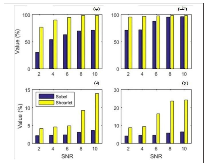
۶ شکل مقایسه‌ی کمی طرح‌واره‌ی شیرلت دوبعدی و پالایه‌ی سوبل با استفاده از آزمایش دسته‌بندی دودویی: الف) ویژگی (ب) دقت (ج) اندازه‌ی F-د) حساسیت برای نسبت‌های سیگنال به نوفه‌ی ۲، ۴، ۶، ۸ و ۱۰. از آنجا که عملگر کنی نتایج کیفی قابل‌قبولی ارائه نداده در محاسبه‌ی کمی از آن استفاده نشده است
