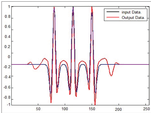
شکل ۵ | ۵ | تداخل سه بازتابنده با یکدیگر (ردلرزه ورودی سیاه‌رنگ و ردلرزه خروجی قرمز رنگ است)
