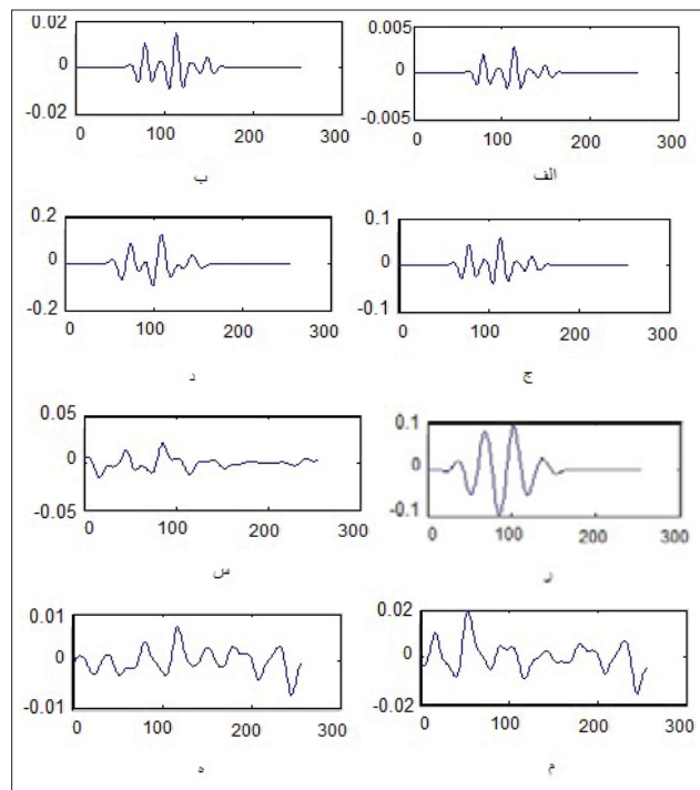
شکل ۴ | ۴ | مشاهده هفت مرحله تجزیه ردلرزه ورودی با تبدیل موجک گسسته پایا از چپ به راست: الف) ردلرزه ورودی. ب) تا ه) مرحله اول تا هفتم تجزیه ردلرزه ورودی
