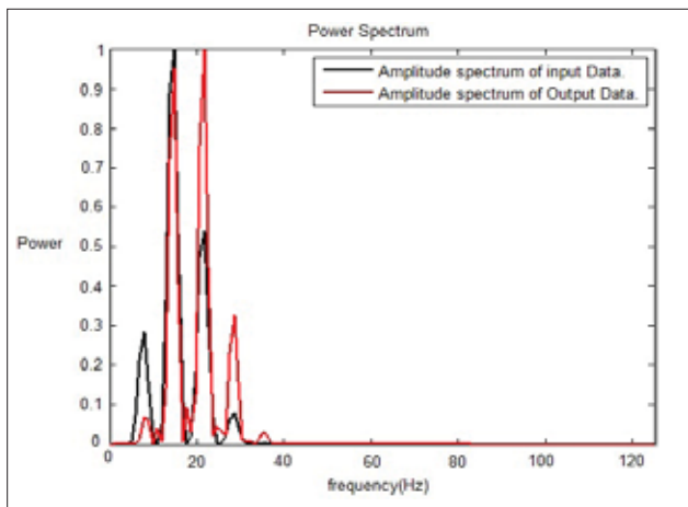
شکل ۶ | ۶ | طیف دامنه که در این طیف ارتقای فرکانسی را نشان می‌دهد (طیف دامنه ورودی سیاه‌رنگ و طیف دامنه خروجی قرمز رنگ است)
